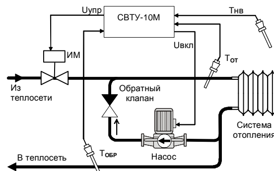
Рис.4 Регулирование температуры на входе контура отопления с коррекцией по T_{нв}
