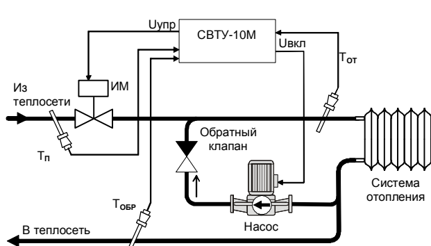
Рис.5 Регулирование температуры на входе контура отопления с ограничением температуры «обратки»
